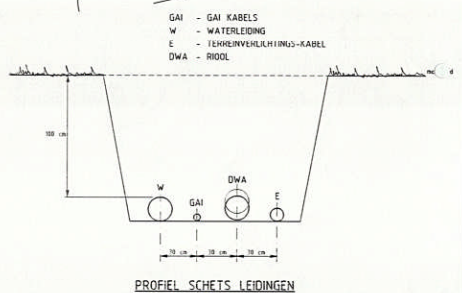
PROFIEL SCHETS LEIDINGEN
